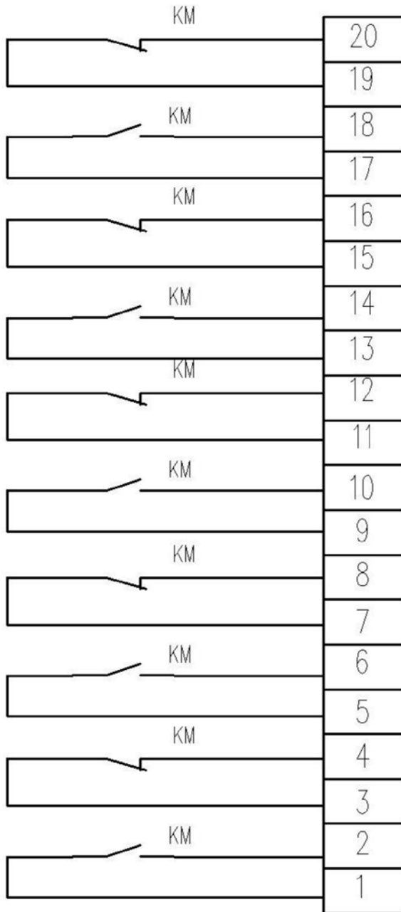
Рисунок 3 - Схема подключения вакуумного контактора с механическим удержанием
