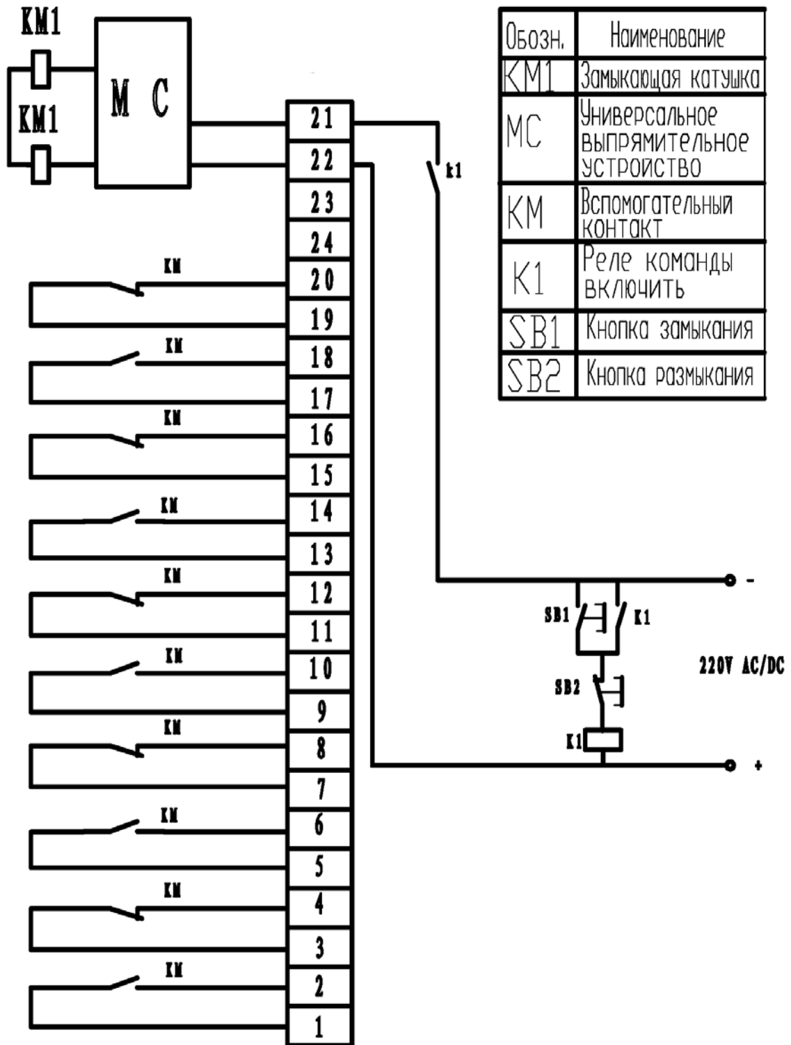
Рисунок 4 - Схема подключения вакуумного контактора с электромагнитным удержанием
