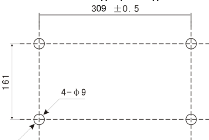
Рисунок 1 - Установочные размеры контактора серии JCZ5
