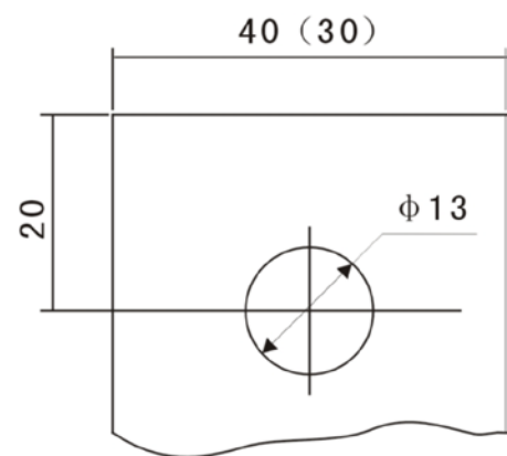
Рисунок 2 – Размеры входных и выходных шин
