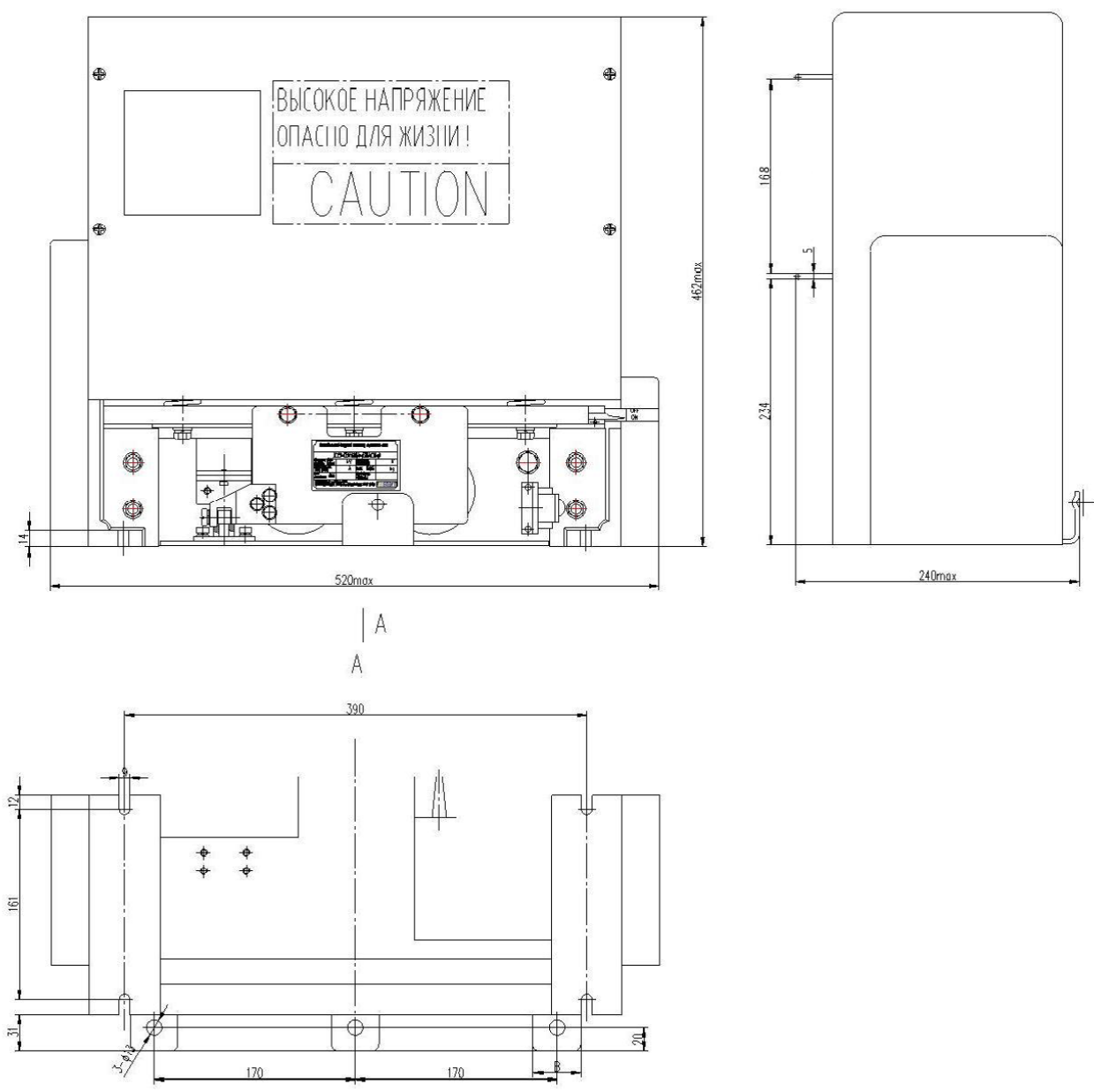
Рисунок 7 – Габаритные размеры контактора
